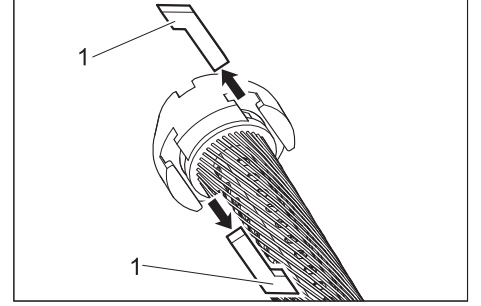
1 Oluk taşı
